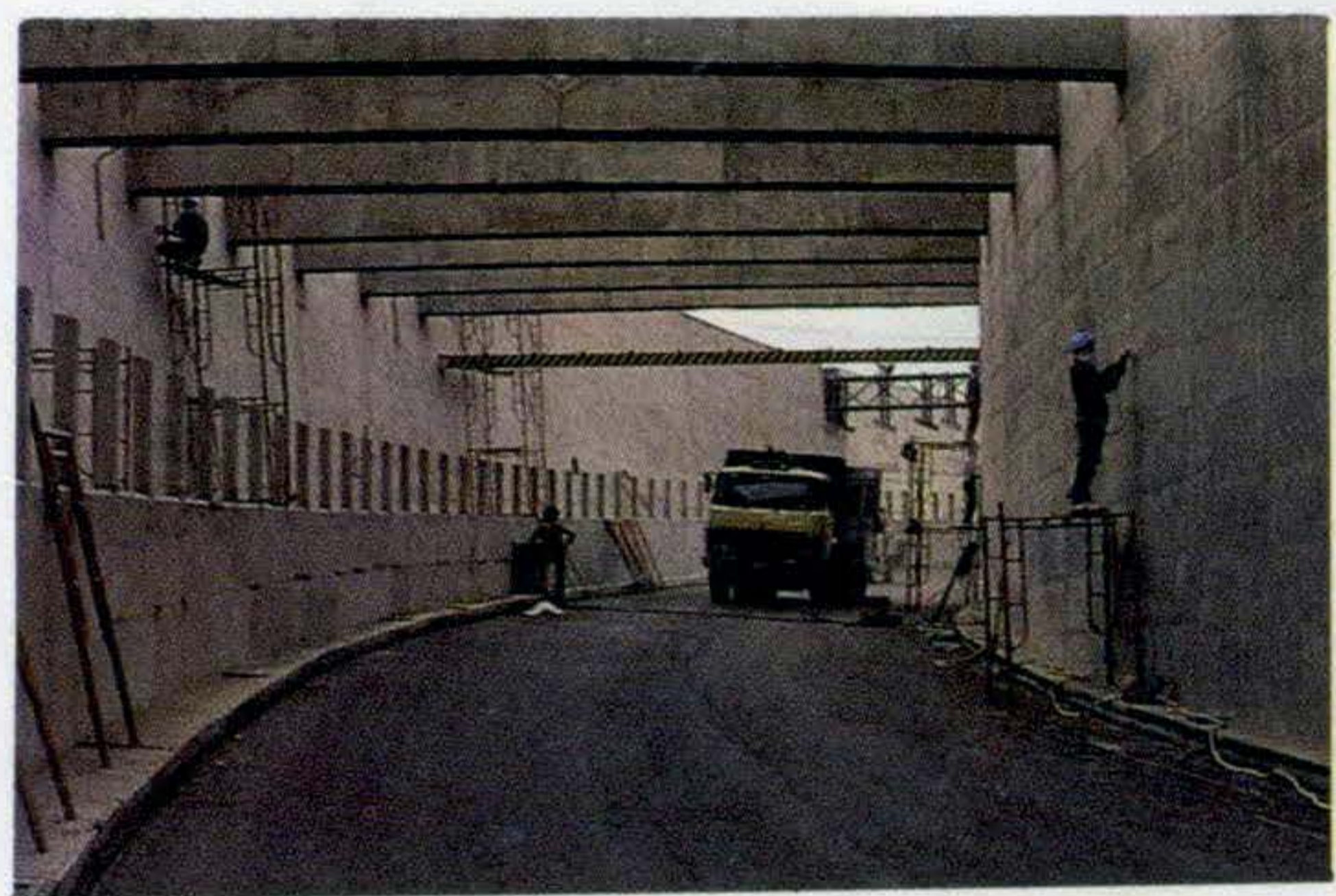
正在趕工中的過港隧道。
