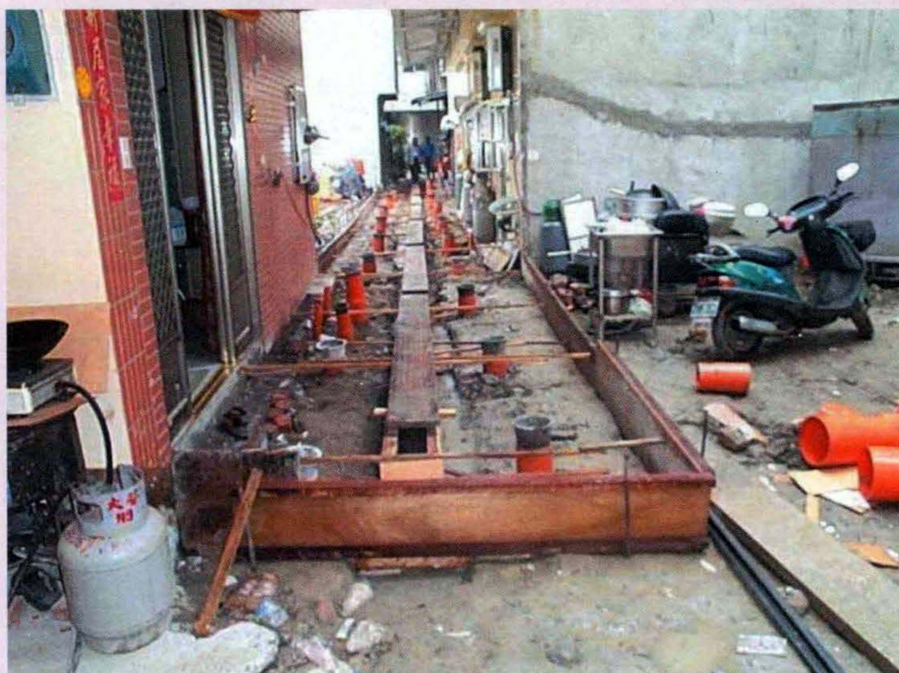
施工中的巷弄，每戶接管完成大約需要2星期時間。 (圖片提供 / 高雄市政府工務局)
